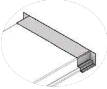
30 AD 200S Bağlantı Örneği 30 AD 200S Connection Example
