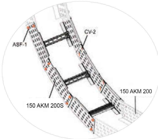
150 AKM 200S Bağlantı Örneği 150 AKM 200S Connection Example
