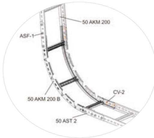
50 AKM 200 B Bağlantı Örneği 50 AKM 200 B Connection Example
