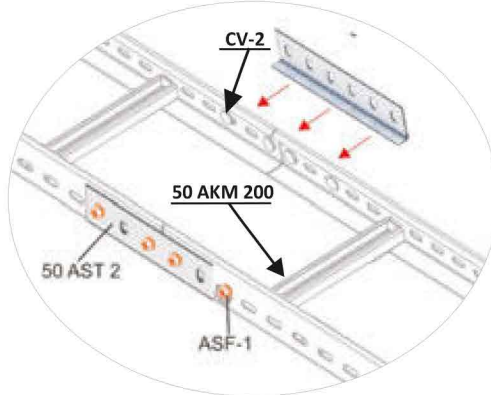
50 AST2 Bağlantı Örneği 50 AST2 Connection Example
