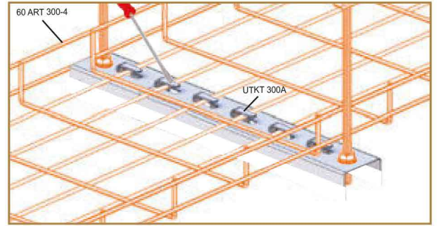
UTKT 300 Bağlantıörneği UTKT 300 Connection Example
