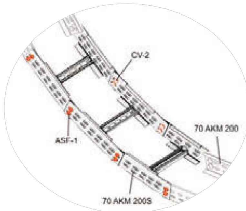
70 AKM 200S Bağlantı Örneği 70 AKM 200S Connection Example
