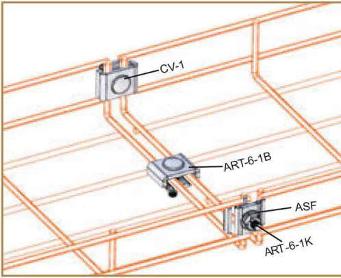
ART-6-1B Bağlantı Örneği
