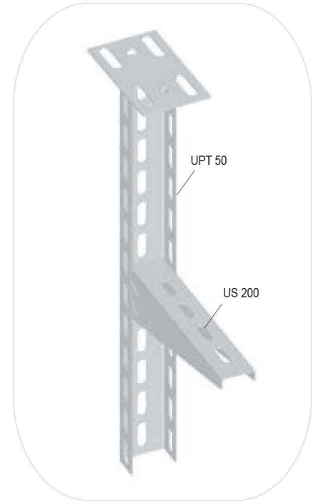
UPT 50 Bağlantı Örneği UPT 50 Connection Example
