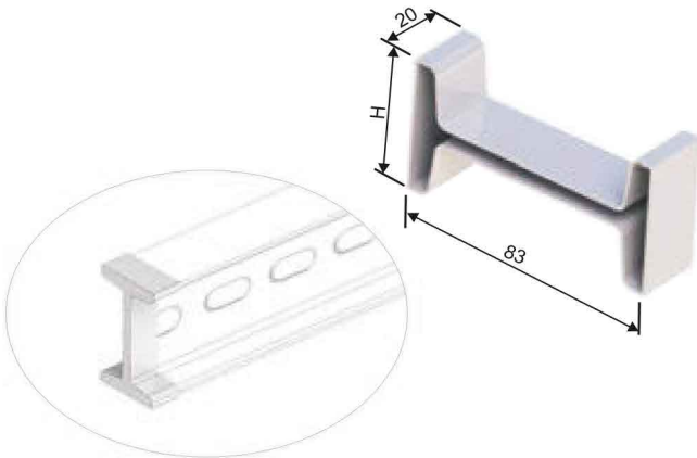
IPS 80 Bağlantı Örneği IPS 80 Connection Example
