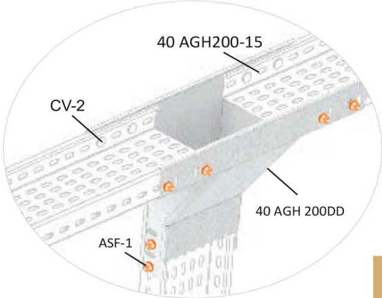
40 AGH 200DD Bağlantı Örneği 40 AGH 200DD Connection Example
