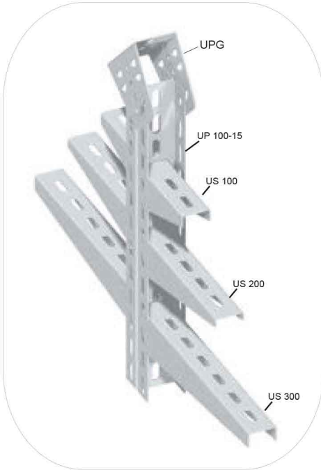
UPG Bağlantı Örneği (Çift U Profil) UPG Connection Example (Double U Profile)
