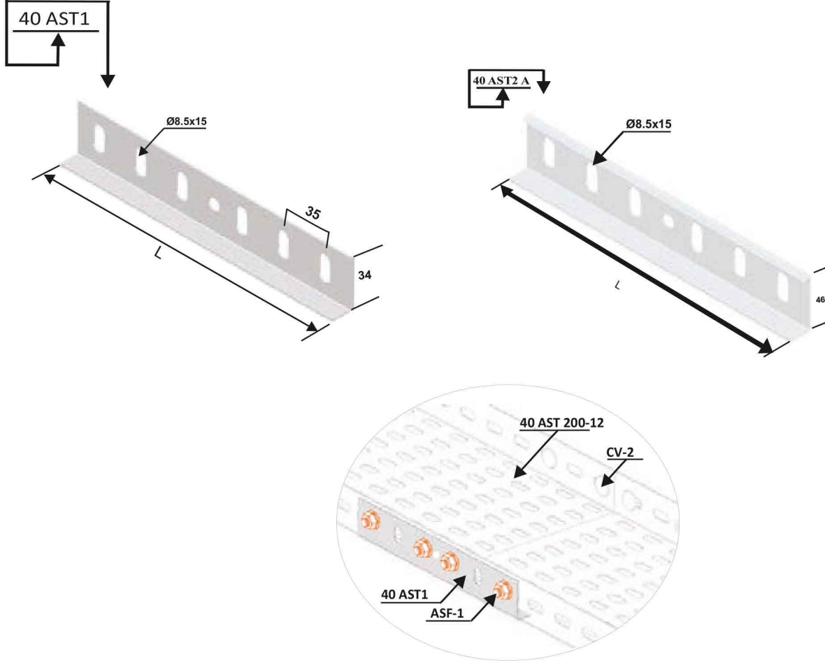
40 AST1 Bağlantı Örneği 40 AST1 Connection Example
