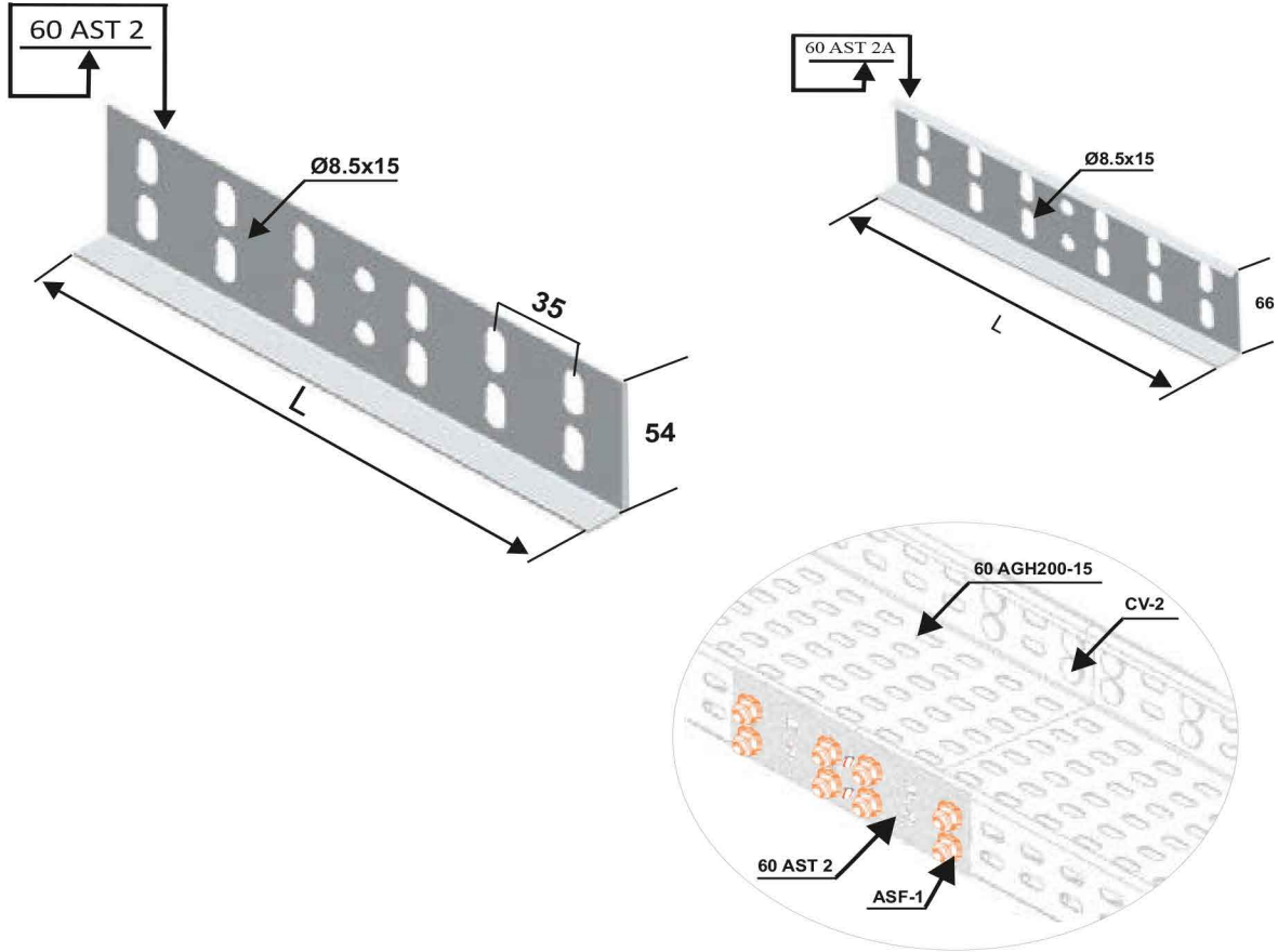
60 AST 2 Bağlantı Örneği 60 AST 2 Connection Example
