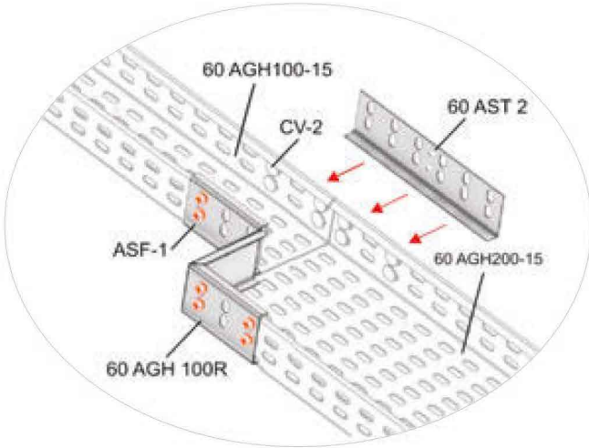
60 AGH 100R Bağlantı Örneği 60 AGH 100R Connection Example
