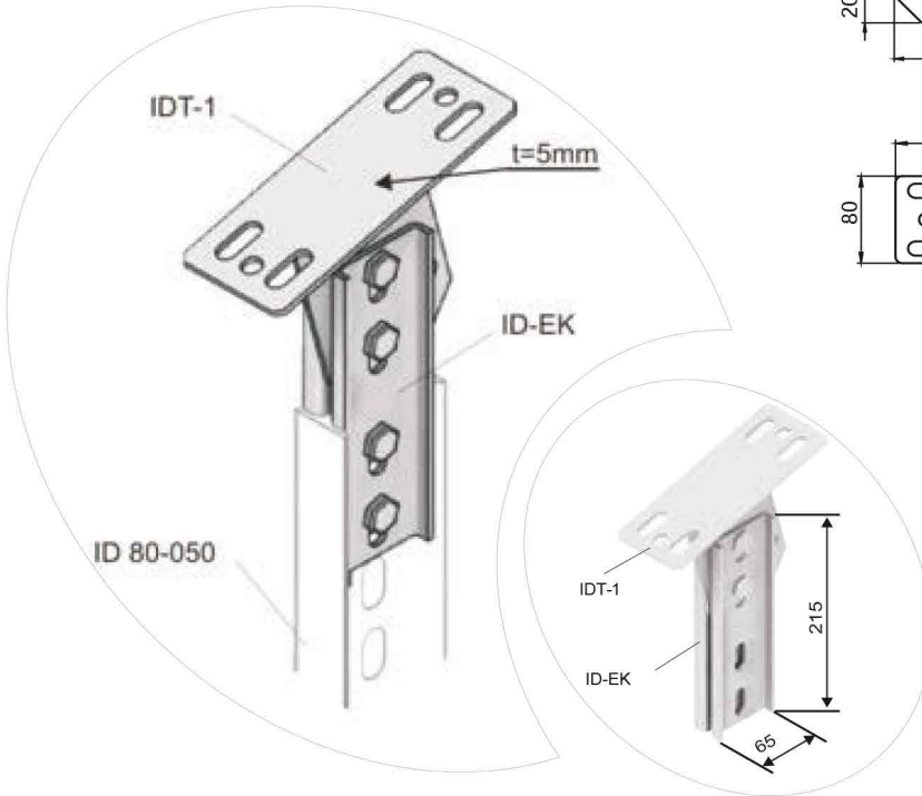
IDT-1 & ID-EK Bağlantı Örneği
