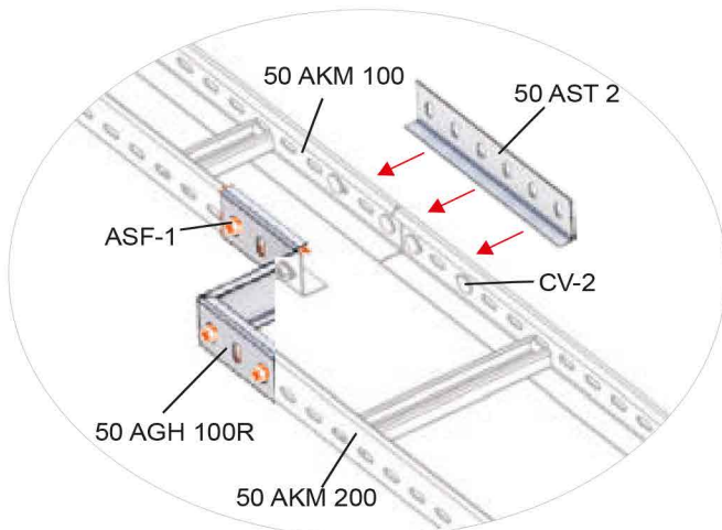
50 AGH 100R Bağlantı Örneği 50 AGH 100R Connection Example
