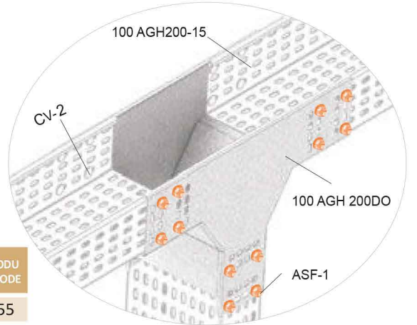
100 AGH 200DO Bağlantı Örneği 100 AGH 200DO Connection Example
