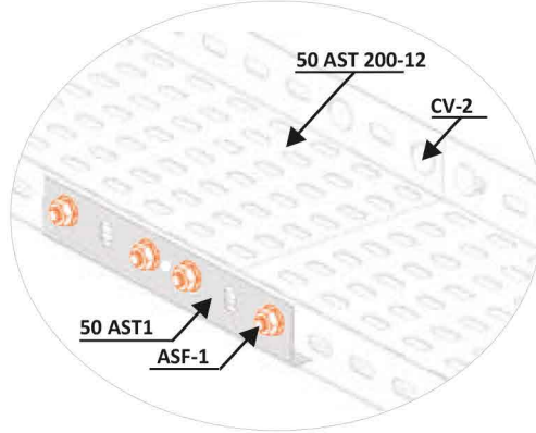
50 AST1 Bağlantı Örneği 50 AST1 Connection Example
