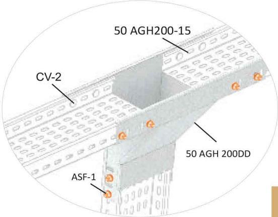
50 AGH 200DD Bağlantı Örneği 50 AGH 200DD Connection Example
