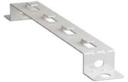
UTKT 300 Bağlantıörneği UTKT 300 Connection Example
