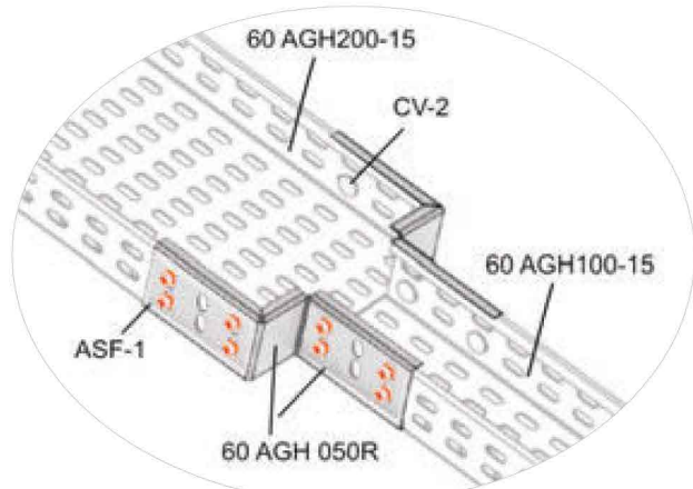
60 AGH 050R Bağlantı Örneği 60 AGH 050R Connection Example
