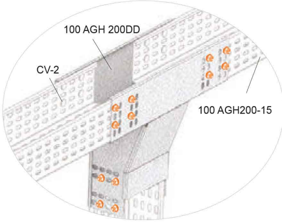
100 AGH 200DD Bağlantı Örneği 100 AGH 200DD Connection Example
