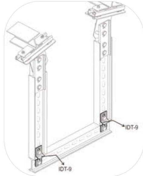
IDT-9 Bağlantı Örneği IDT-9 Connection example
