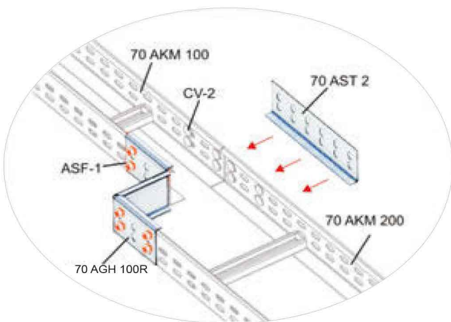
70 AGH 100R Bağlantı Örneği 70 AGH 100R Connection Example
