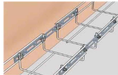
Mesafe ayarlı bağlantı / Connection from the distance
