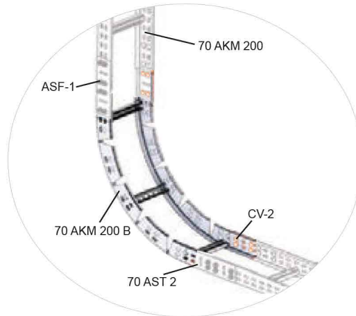
70 AKM 200 B Bağlantı Örneği 70 AKM 200 B Connection Example
