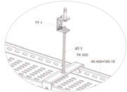
TT 1 Bağlantı Örneği TT 1 Connection Example
