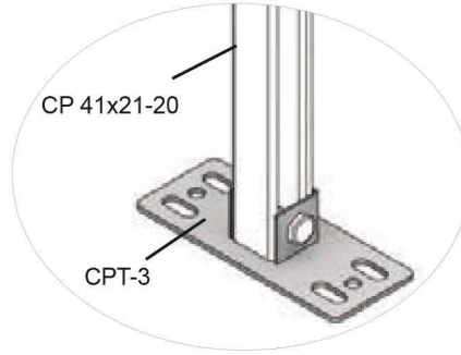
CPT-3 Bağlantı Örneği CPT-3 Connection Example
