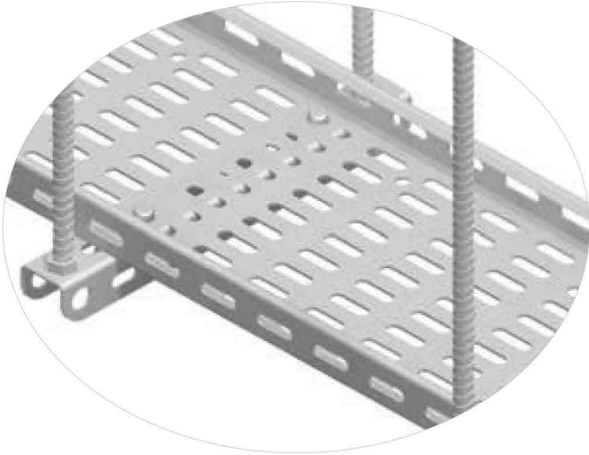
UTK 200 Bağlantıörneđi UTK 200 Connection Example
