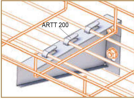
ARTT 200 Bağlantıörneği ARTT 200 Connection Example
