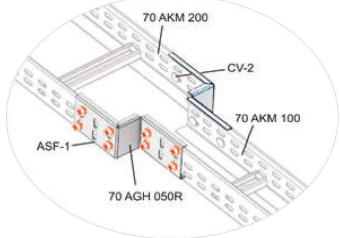
70 AGH 050R Bağlantı Örneği 70 AGH 050R Connection Example
