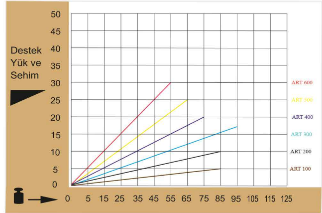
Kaynaksız Duvar Konsolları Yük ve Sehim Grafiği
