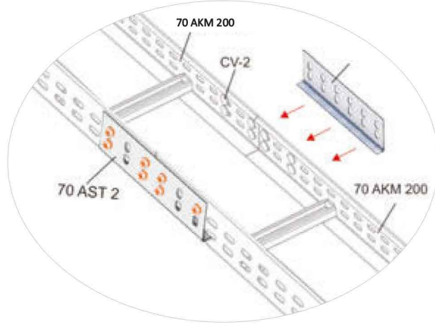
70 AST2 Bağlantı Örneği 70 AST2 Connection Example
