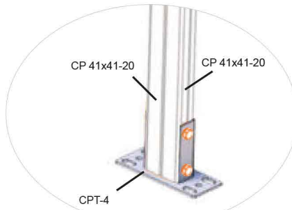
CPT-4 Bağlantı Örneği CPT-4 Connection Example
