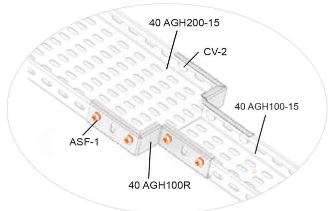
40 AGH 200-15 Bağlantı Örneği 40 AGH 200-15 Connection Example
