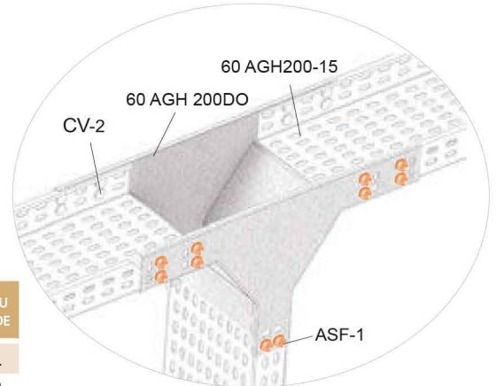
60 AGH 200DO Bağlantı Örneği 60 AGH 200DO Connection Example
