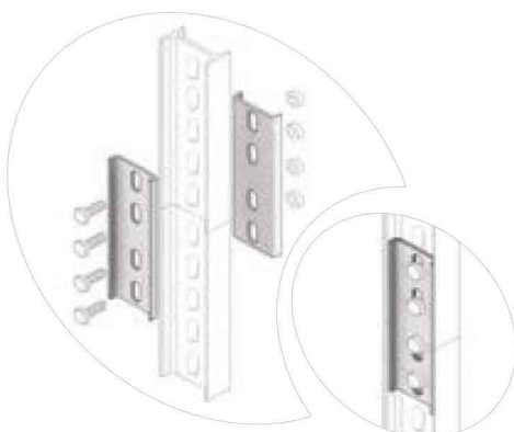
ID-EK Bağlantı Örneği ID-EK Connection example
