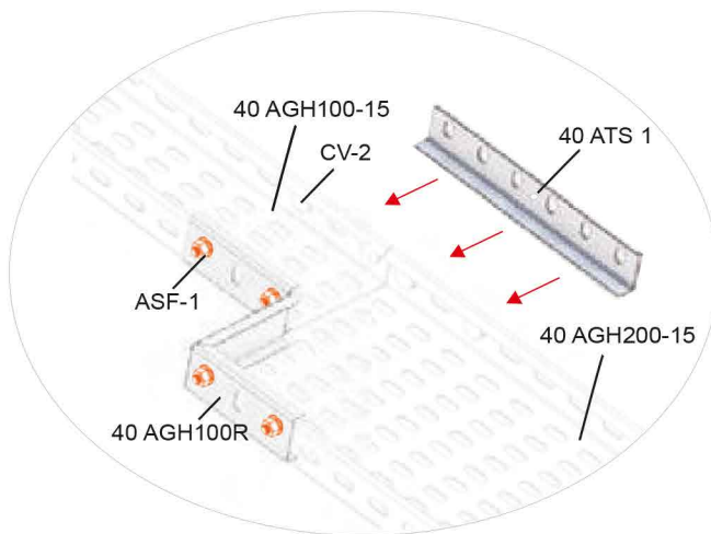
40 AGH 100R Bağlantı Örneği 40 AGH 100 R Connection Example
