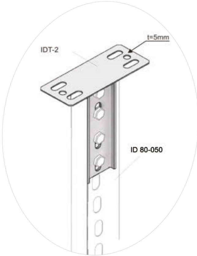
IDT-2 Bağlantı Örneği
