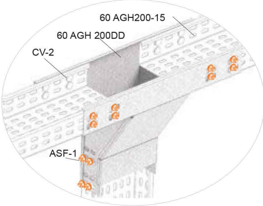
60 AGH 200DD Bağlantı Örneği 60 AGH 200DD Connection Example
