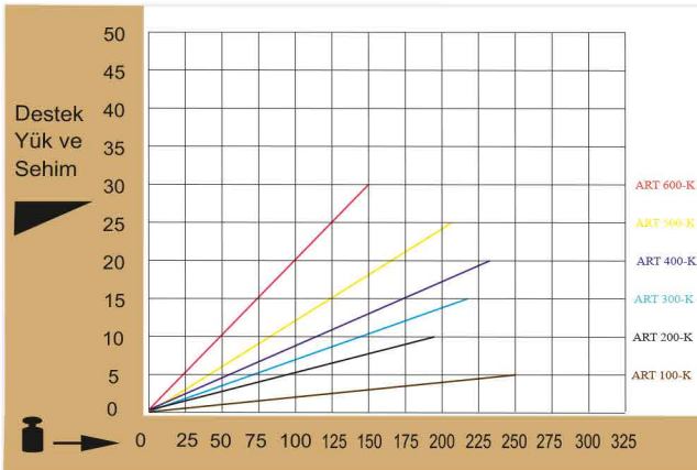
Kaynaklı Duvar Konsolları Yük ve Sehim Grafiği
