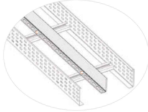
100 AKM 15S Bağlantı Örneği 100 AKM 15S Connection Example
