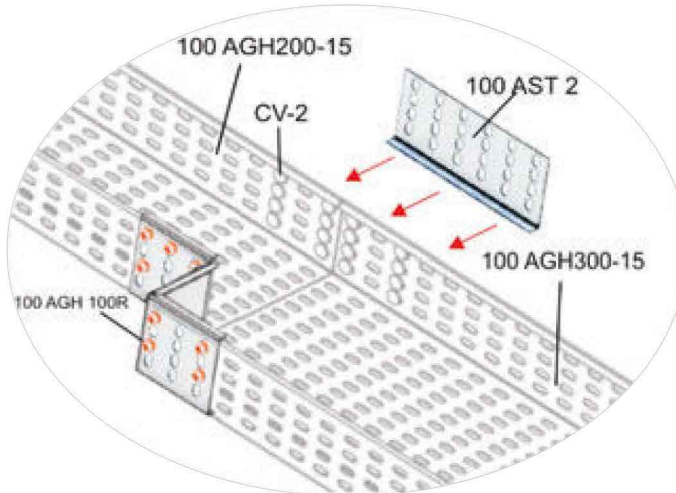
100 AGH 100R Bağlantı Örneği 100 AGH 100R Connection Example
