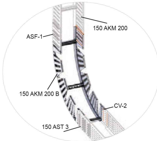
150 AKM 200 B Bağlantı Örneği 150 AKM 200 B Connection Example
