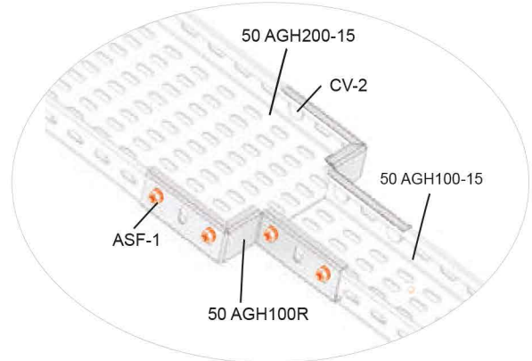
50 AGH 100R Bağlantı Örneği 50 AGH 100R Connection Example
