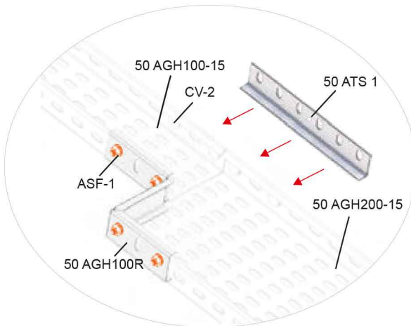
50 AGH 100R Bağlantı Örneği 50 AGH 100 R Connection Example
