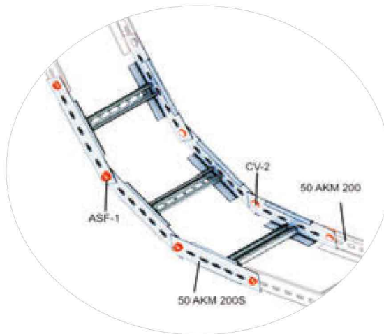
50 AKM 200S Bağlantı Örneği 50 AKM 200S Connection Example
