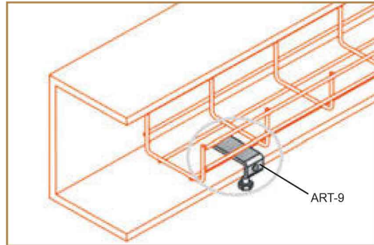
ART-9 Bağlantı Örneği
