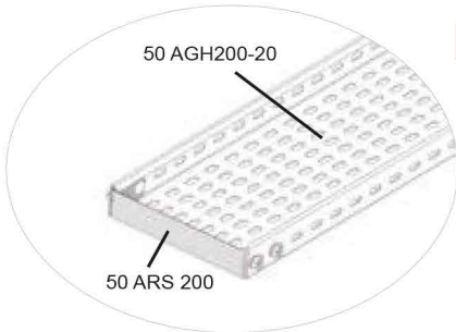
50 ARS 200 Bağlantı Örneği 50 ARS 200 Connection Example
