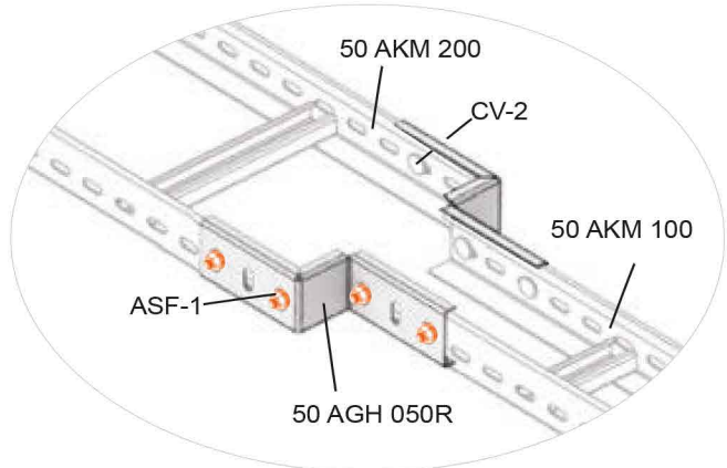
50 AGH 050R Bağlantı Örneği 50 AGH 050R Connection Example
