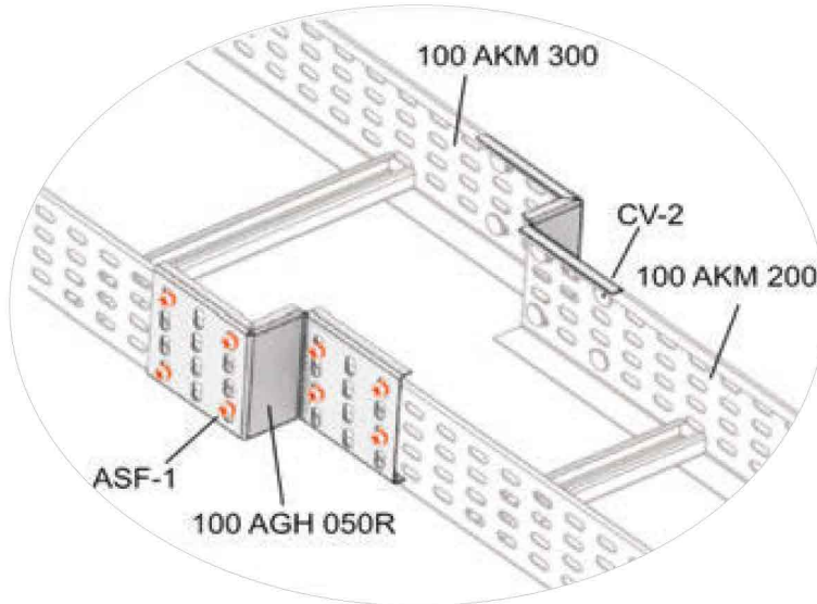
100 AGH 050R Bağlantı Örneği 100 AGH 050R Connection Example
