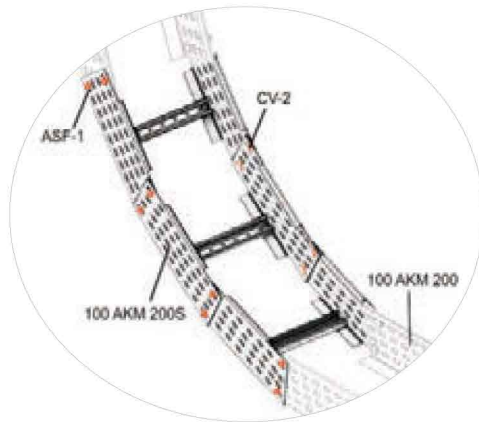
100 AKM 200S Bağlantı Örneği 100 AKM 200S Connection Example
