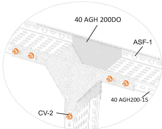
40 AGH 200DO Bağlantı Örneği 40 AGH 200DO Connection Example
