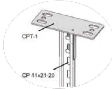
CPT-1 Bağlantı Örneği CPT-1 Connection Example
