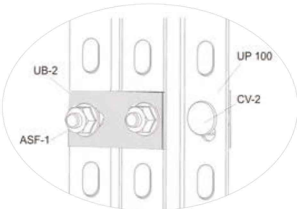
UB-2 Bağlantı Örneği UB-2 Connection Example
