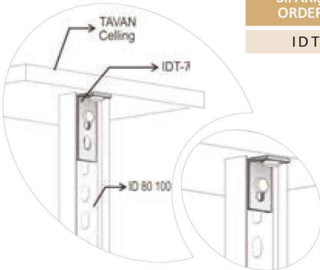
IDT-7 Bağlantı Örneği IDT-7 Connection Example
