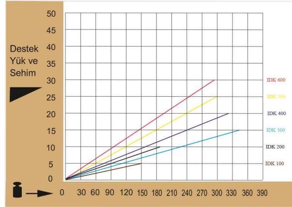
I Destek KonsollarıYük ve Sehim Grafiği
