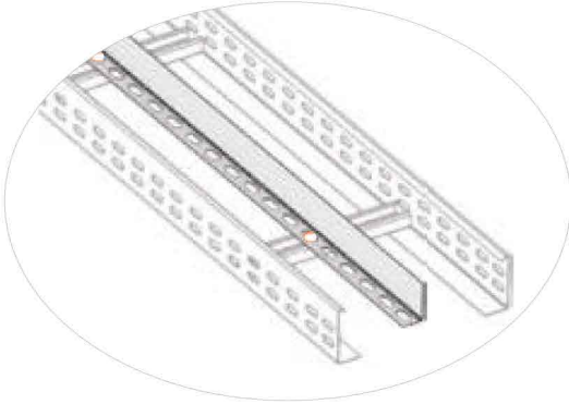
70 AKM 13S Bağlantı Örneği 70 AKM 13S Connection Example
