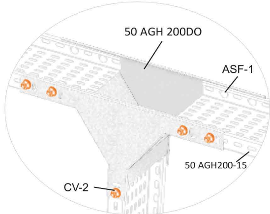
50 AGH 200DO Bağlantı Örneği 50 AGH 200DO Connection Example
