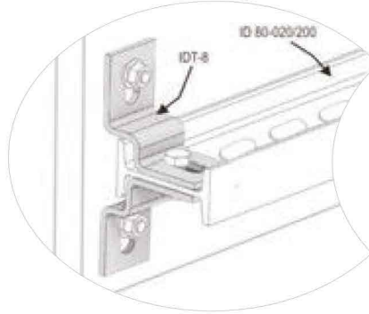
IDT-8 Bağlantı Örneği IDT-8 Connection example
