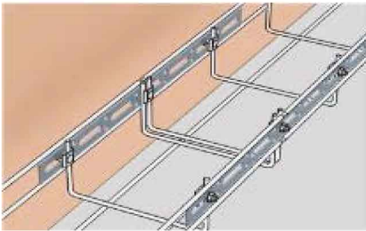
Düz Bağlantı / Standard Connection
