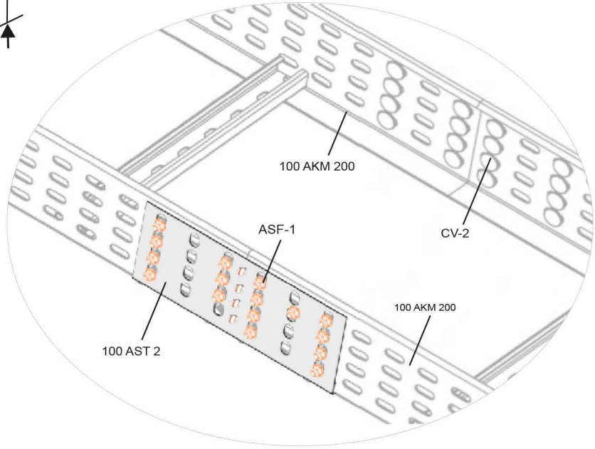
100 AST 2 Bağlantı Örneği 100 AST 2 Connection Example
