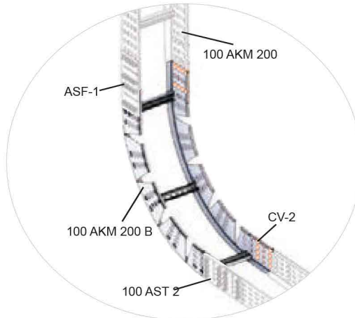
100 AKM 200 B Bağlantı Örneği 100 AKM 200 B Connection Example
