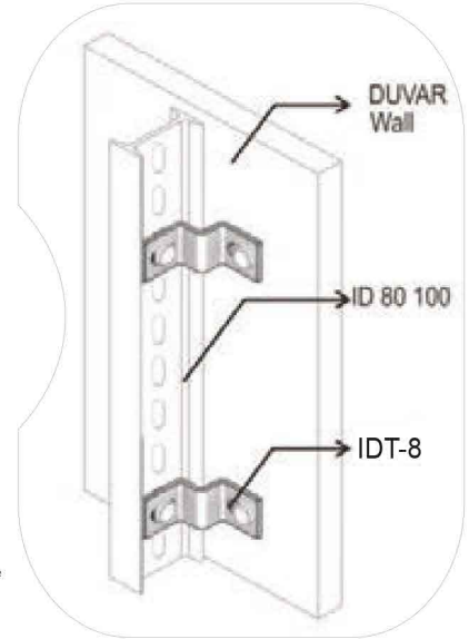
IDT-8 Bağlantı Örneği IDT-8 Connection example
