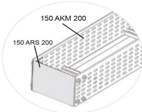
150 ARS 200 Bađlantı Örneđi 150 ARS 200 Connection Example
