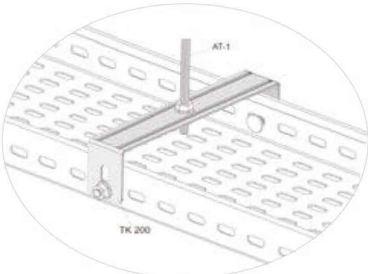
TK 200 Bağlantı Örneği TK 200 Connection Example
