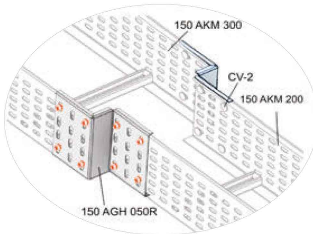
150 AGH 050R Bağlantı Örneği 150 AGH 050R Connection Example
